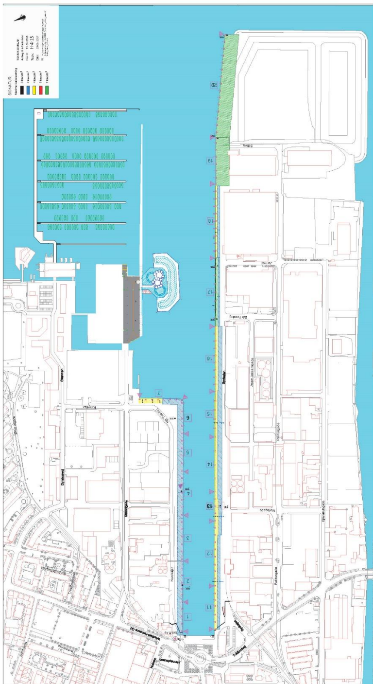
Fig. Kort over kajbelastning på Vejle Erhvervshavn
